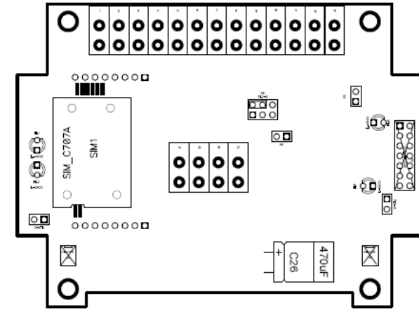
Рис. 7.1 Схема клеммников счетчика
